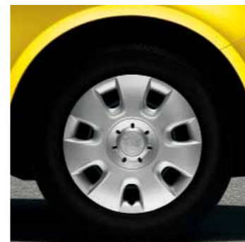
Velkoplošné kryty Draco pro kola 5,0J x 14", čtyřdílná sada (CDB 700 003)
